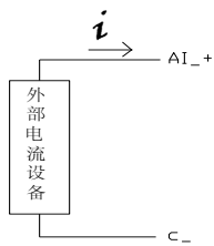
XL-E4AD2DA 电流输入侧接线如下图所示：
