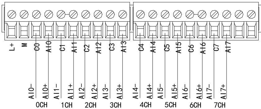
XL-E8AD-A-S 电流输入侧接线如下图所示：
