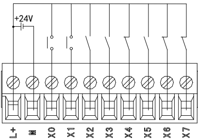
开关按钮接线图示例
