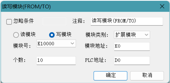
(b) 写模块
