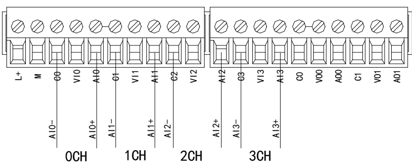
XL-E4AD2DA 电流输入侧接线如下图所示：
