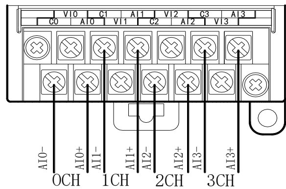
XD-E4AD 电流输入侧接线如下图所示：
