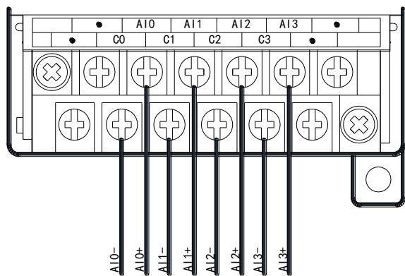
XD-E8AD 电流输入侧接线如下图所示：
