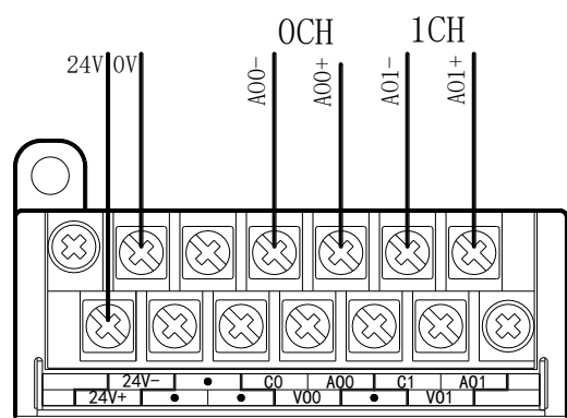
XD-E4DA 电流输出侧接线如下图所示：
