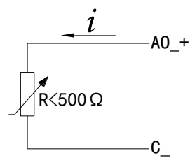
XD-E4DA 电流输出侧接线如下图所示：
