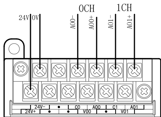
XD-E2DA 电流输出侧接线如下图所示：
