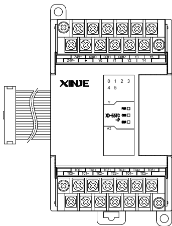
XD-E6TC-P/XD-E6TC-P-H/XD-E2TC-P 温度 PID 控制模块，对 6/2 点热电偶温度信号进行处理，并把它们传输到 PLC 主单元。
