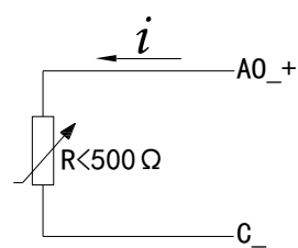
XD-E2DA 电流输出侧接线如下图所示：
