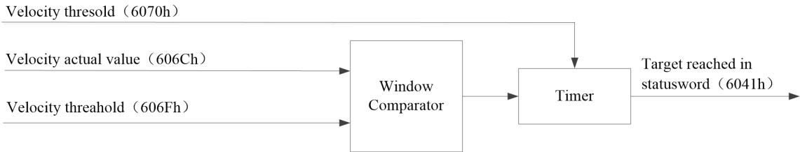
< Speed（functional overview）>
