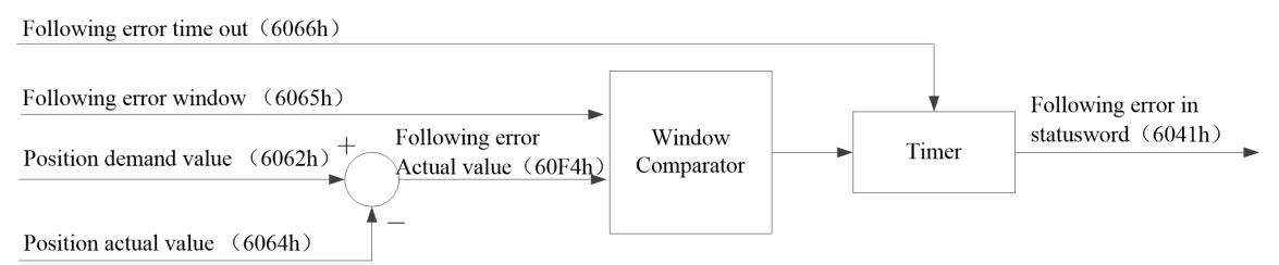
跟随误差功能示意图
