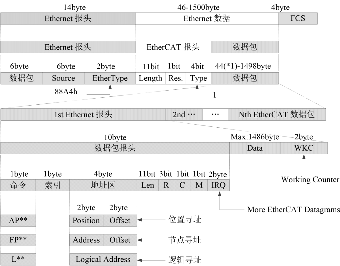
EtherNet/EtherCAT 帧结构
