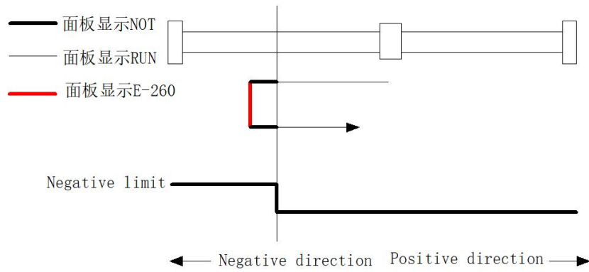
情况2：在轴减速停止完成之前，触碰正向限位开关
